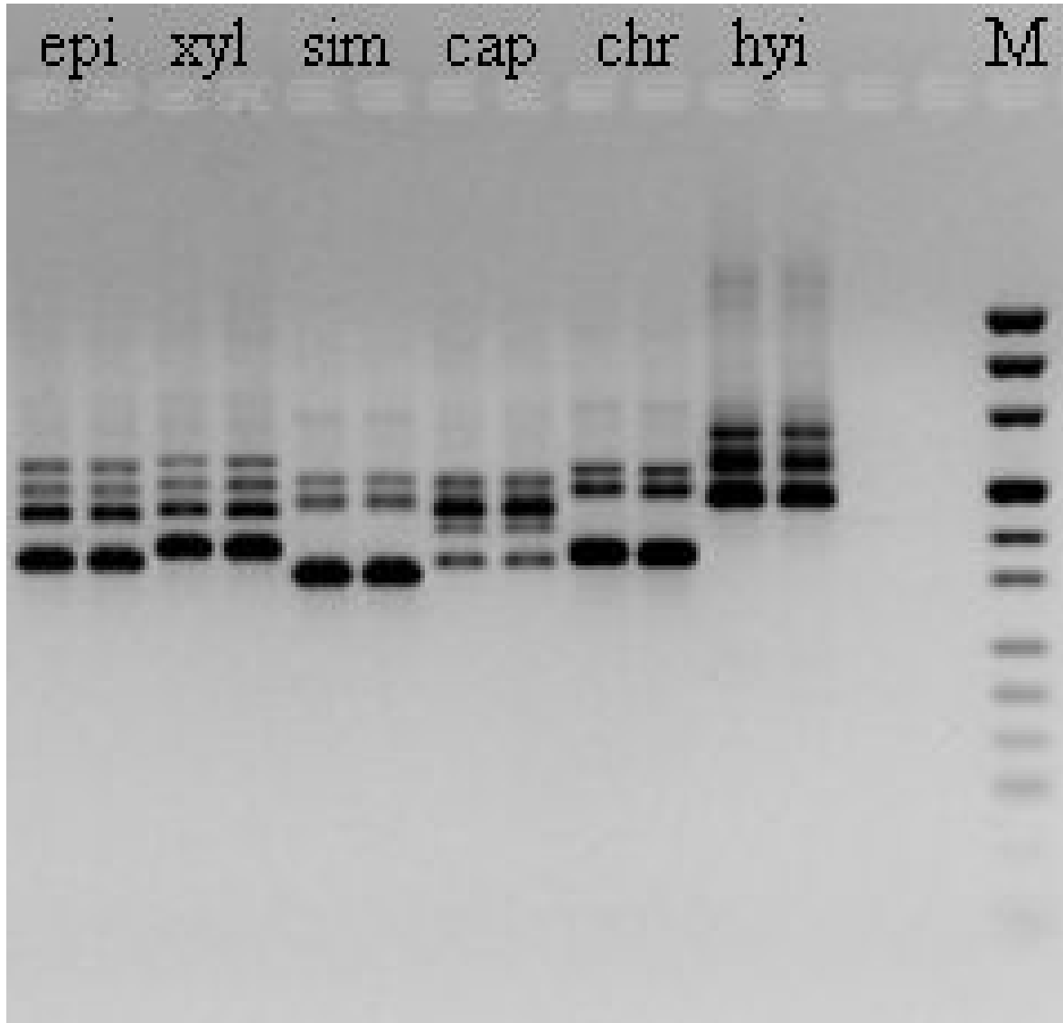
Abb. 3: Charakteristische Bandenmuster nach ITS-PCR, epi: S. epidermidis , xyl: S. xyloso , sim: S. simulans , cap: S. caprae , chr: S. chromogenes , hyi: S. hyicus , M: Größenmarker – Characteristic pattern from ITS-PCR, epi: S. epidermidis , xyl: S. xyloso , sim: S. simulans , cap: S. caprae , chr: S. chromogenes , hyi: S. hyicus , M: molecular weight marker
